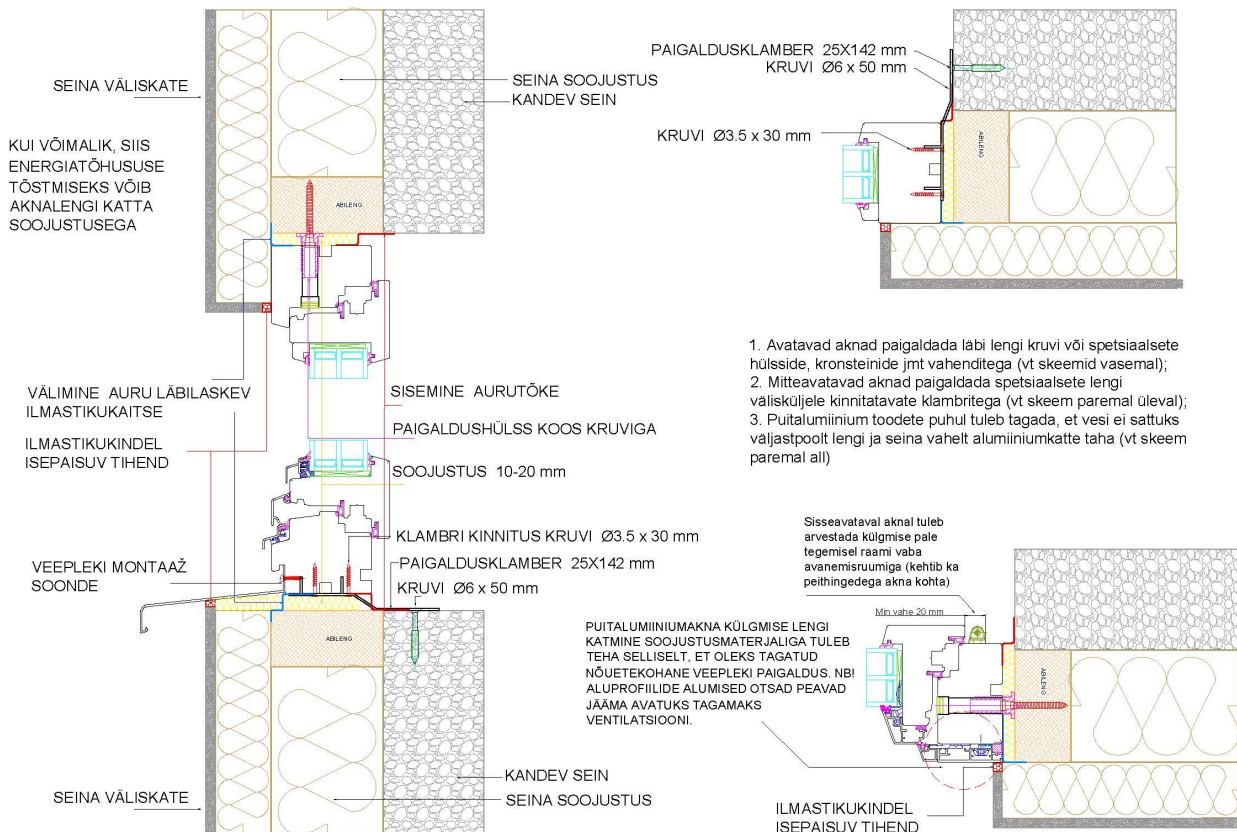
Joonis 6. Sisseavatavad DK22 aknad, rõduksed ja liikandused
