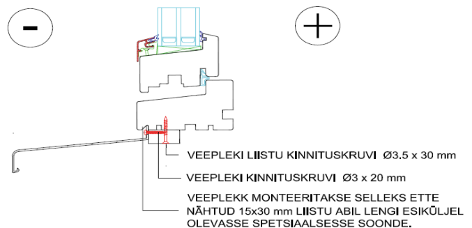
Joonis 3. Väljaavatava akna veepleki kinnitus 15x30 mm liistu abil (välja avatava akna näitel)
