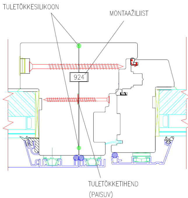
Joonis 13. SW14 tuletõkke akande leng-lengi ühendus (illustreeritud SW14 puitalumiinium tuletõkkeakna näitel)
