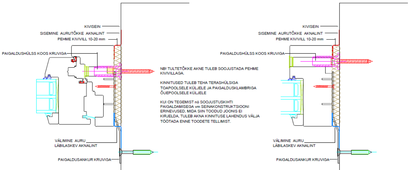
Joonis 10. SW14 tuletõkkeakna paigaldus (NB! joonisel on illustreeritud tavaklaasiga SW14 akent ja ei näidata tuletõkketihendeid jmt konfidentsiaalset informatsiooni)
