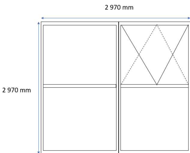
Joonis 12. SW14 tuletõkkehendega on võimalik konstrueerida nn moodulseinasid—mõõdud ja lahendused tuleb täpsustada tootjaga enne toodete tellimist.
