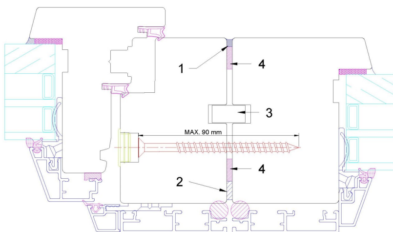
Joonis 12. SW14 tuletõkkehendega on võimalik konstrueerida nn moodulseinasid—mõõdud ja lahendused tuleb täpsustada tootjaga enne toodete tellimist.
