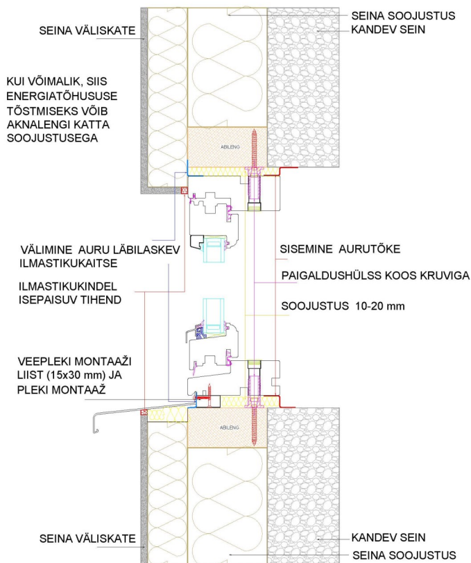
Joonis 4. Viking21 väljaavatava akna paigaldusskeemid
